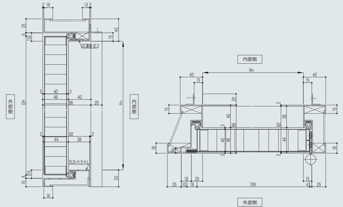
B对震(戸先目板一体型)
