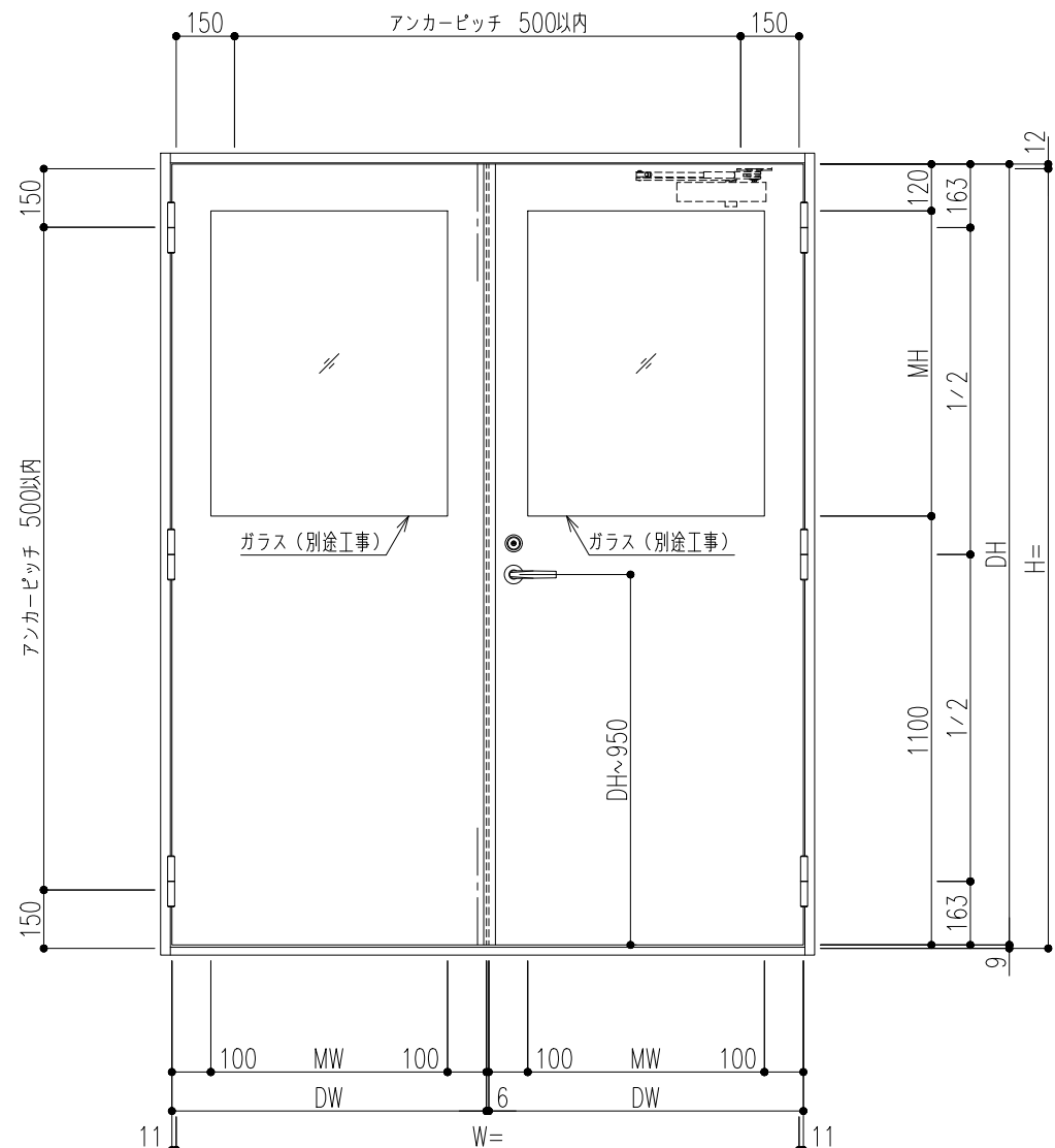
外部側観図
