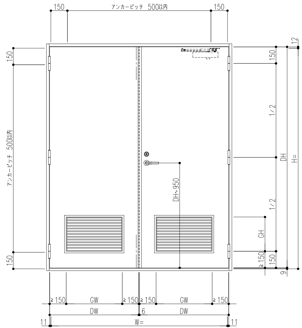
外部側観図
