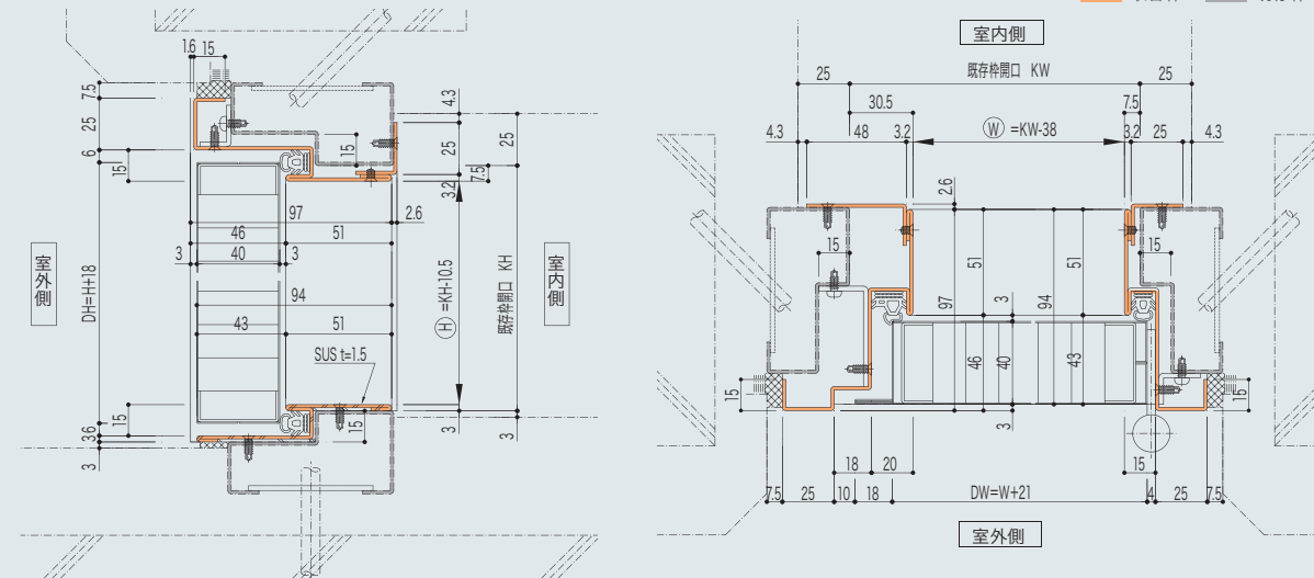
カバー工法 B対震タイプ(内付け納まり)
