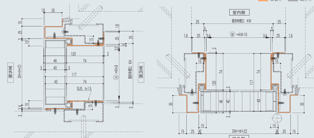
持出し工法(外付け納まり)
