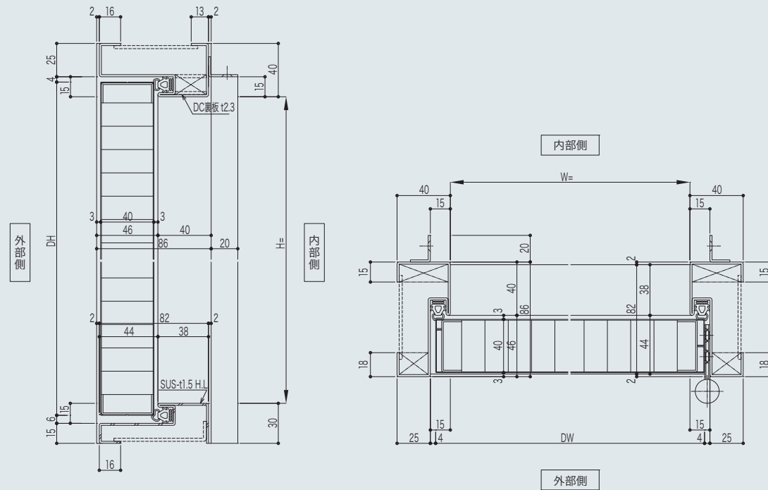
標準断面
