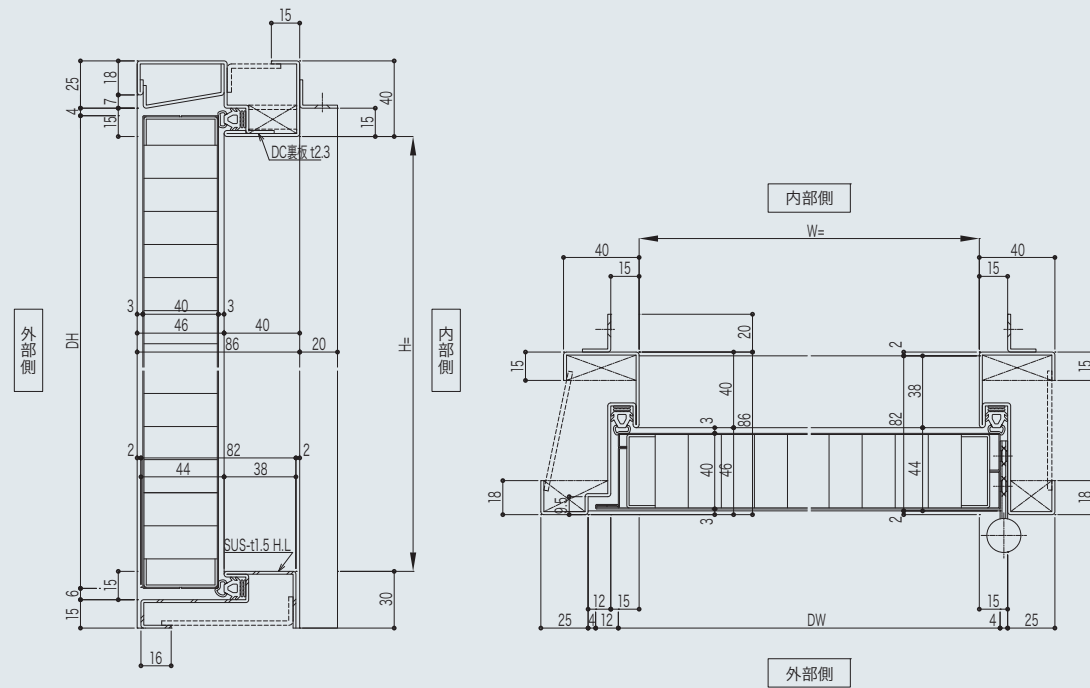
A対震(戸先目板一体)
