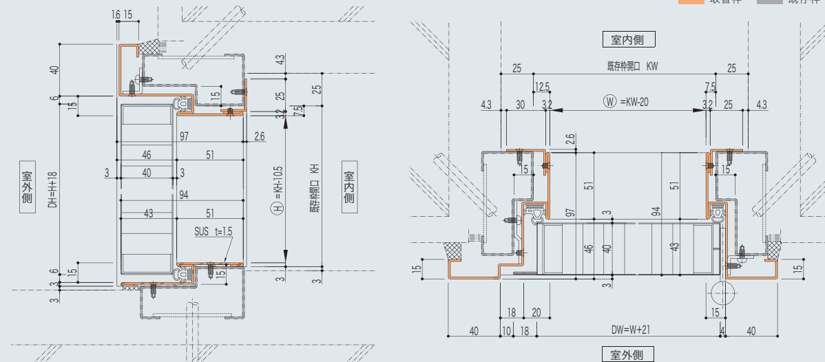
カバー工法 B対震タイプ(外付け納まり)
