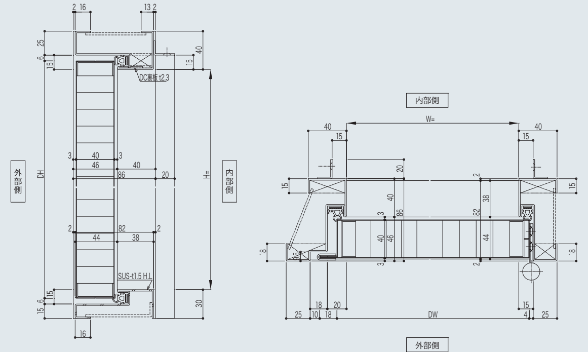
B対震(戸先目板一体型)
