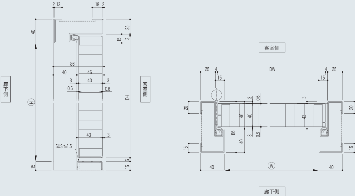
ホテルドア 枠見込み86mm(参考断面1)
